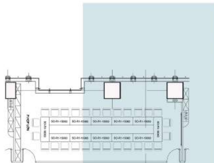
MẶT BẰNG BỐ TRÍ PHÒNG HỌP LỚN
