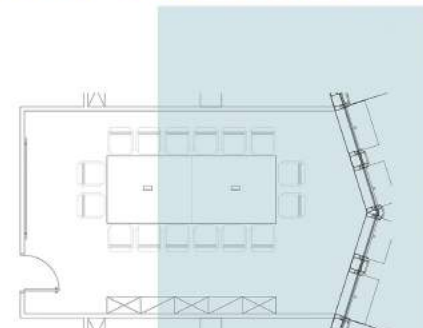
MẶT BẰNG BỐ TRÍ PHÒNG HỌP NHỎ
